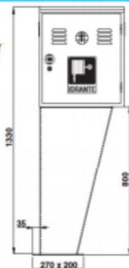
Ingombri di cassetta TEXAS su piantana
